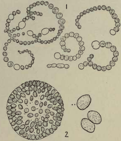
Fig. 479.—Blanket-weed
