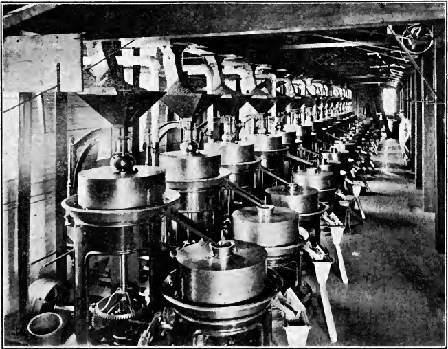
FIG. 42. — Grinding Cocoa.
