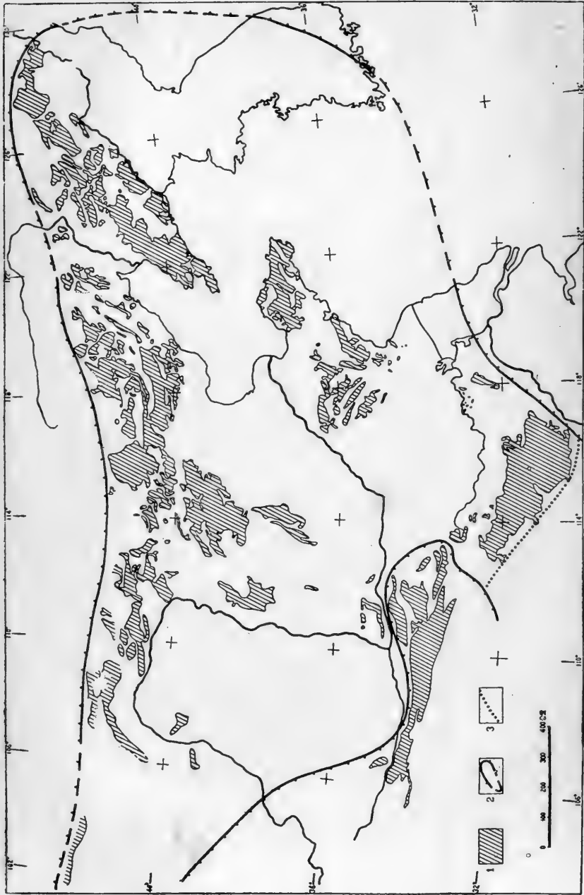
圖3 中朝地台與塞武紀前地層的分佈 1. 塞武紀前地層露頭 2. 中朝地台的範圍 3. 中朝地台南北部的分界
