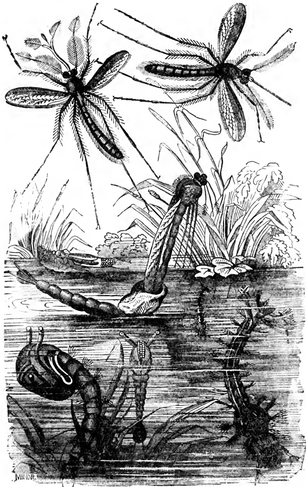
Fig. 4.—GNATS.
