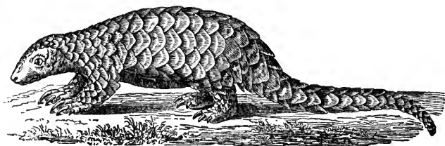
Fig. 9.—THE MANIS.
