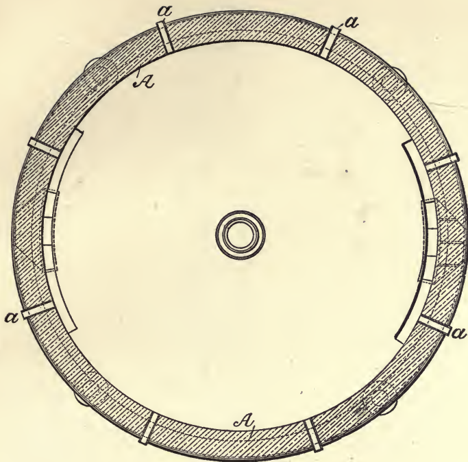
FIG. 85.—Plan.
