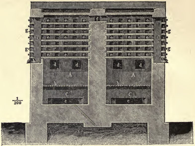
Longitudinal Section.
