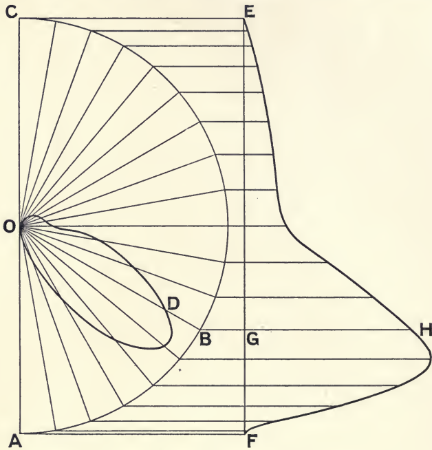
FIG. 110.—ROUSSEAU'S DIAGRAM.
