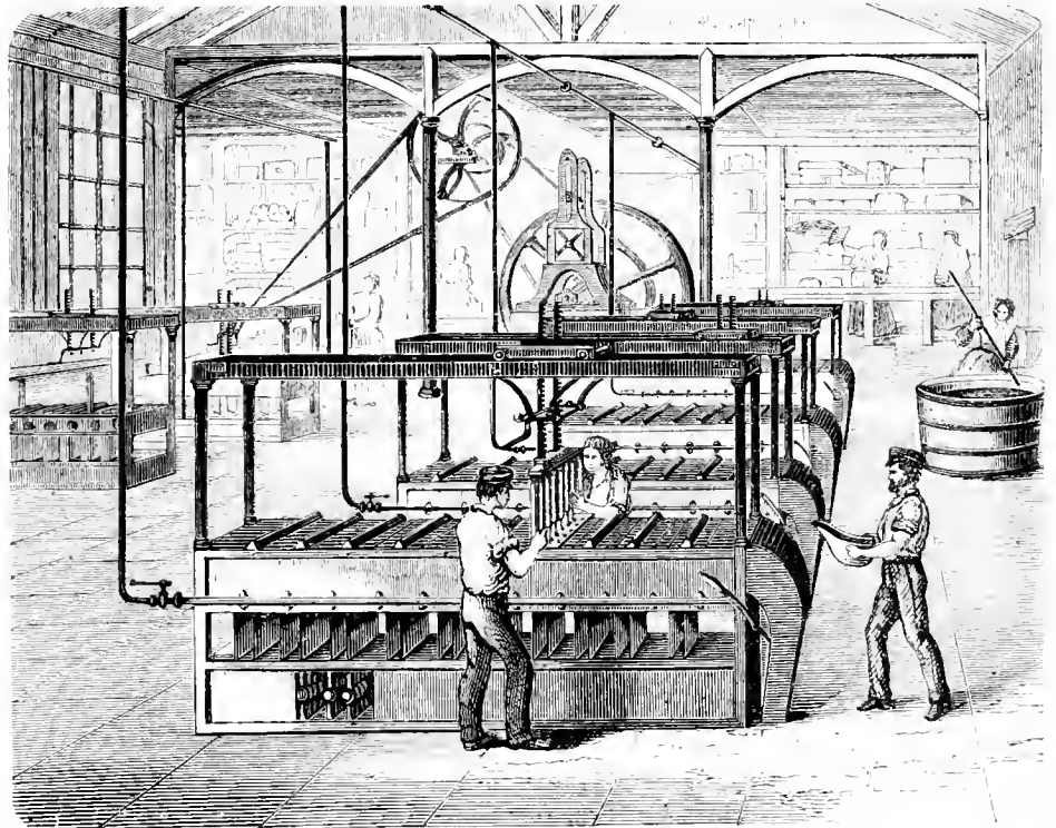
Ar. 3692. Kerzengießmaschine von Alorgau.
