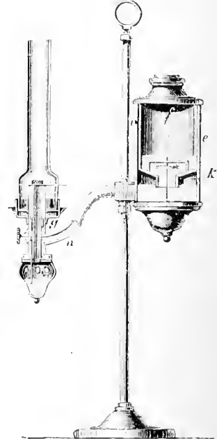
Nr. 3904 Schilde Lampe.
