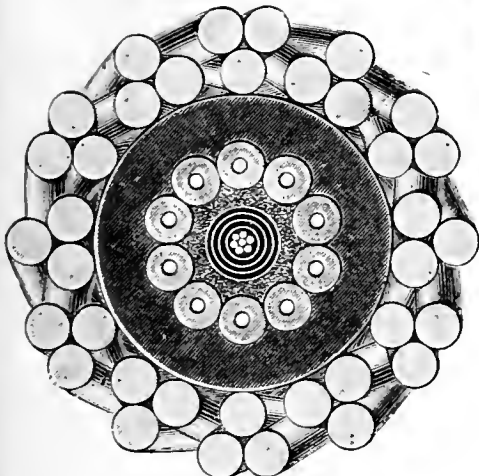
Nr. 3583. Atlantisches Küstenskabel von 1867.
