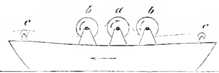
Nr. 3696. Prinzip der Kettenschiffahrt.
