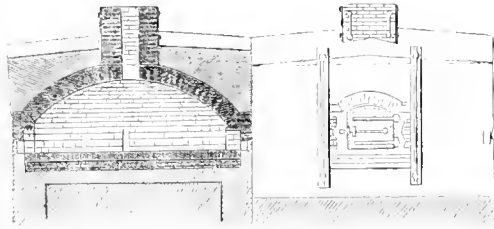
No. 3734 Ofen zum Koks-brennen.
