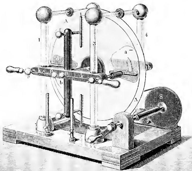
No. 3172. Influenzmaschine von Holz. (Vorderansicht)
