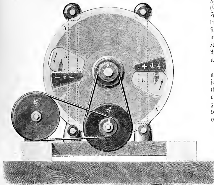
Fig. 3173. Inducentelektrismaschine von Holtz. (Rückansicht.)
