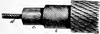
Nr. 3579. Atlantisches Kabel von 1857. a Schale aus Eisendrähten, b Mantel, c Guttapercha- hülle, d Leitungsstrang.
