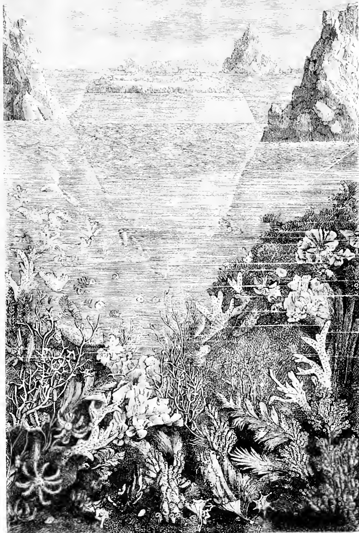
Nr 3737. Aufbau von Koralleninseln (Motten) in der Südsee.
