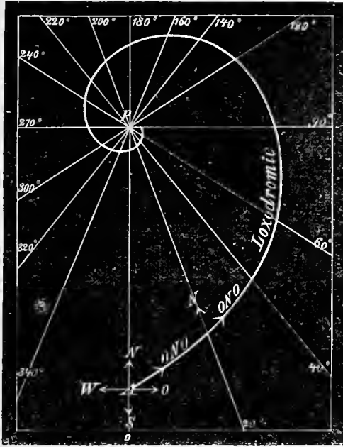
Nr. 4021. Loxodromie.
