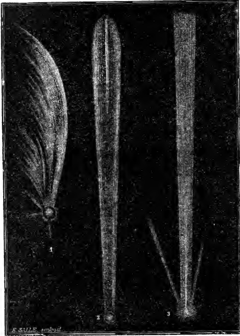
Nr. 3742 3743 3744 3742 Komet von 1577 nach den Beobachtungen von Cornelius Gemma. 3743 Komet von 1689, nach J. C. Sturm. 3744 Komet von 1769.
