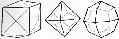
Nr. 3448—3450. Ikoetetraeder.
