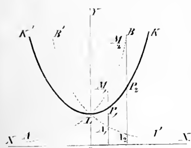
Nr. 3695. Kettenlinie.
