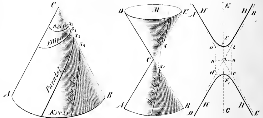
Nr. 3680. Kegelschnitte.
