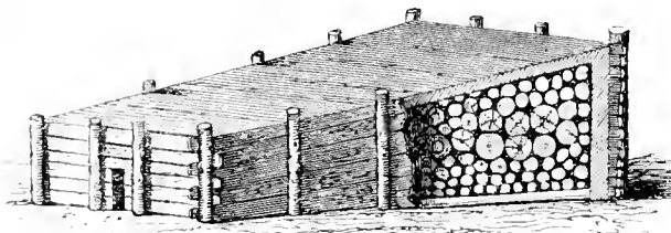
No. 3735. Kohlenweiler, sog. liegendes Werk.
