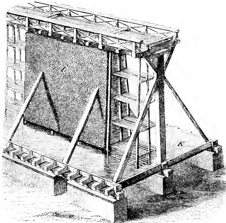
Nr. 3731. Gradirhaus.
