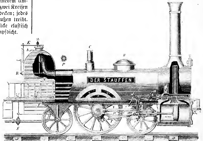
Nr. 495. Seitenansicht einer Lokomotive zur Erläuterung der Hauptbestandtheile.
