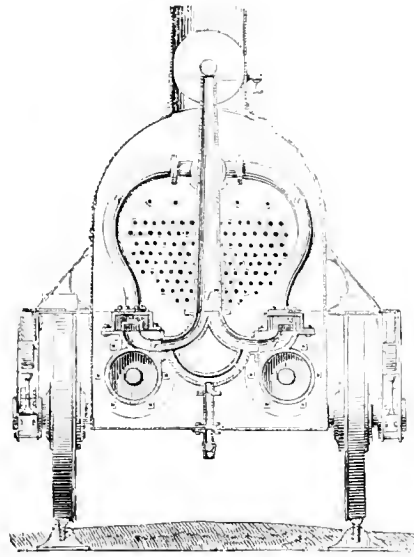
Nr. 4003. Lokomotive. Vorderansicht mit durchschnittenem Kesselraum.
