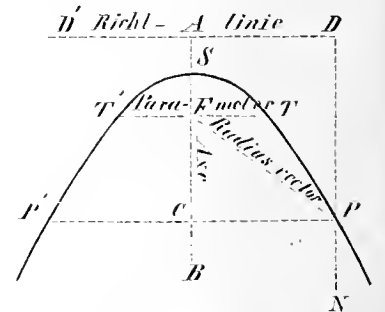
Nr. 3683. Parabel.
