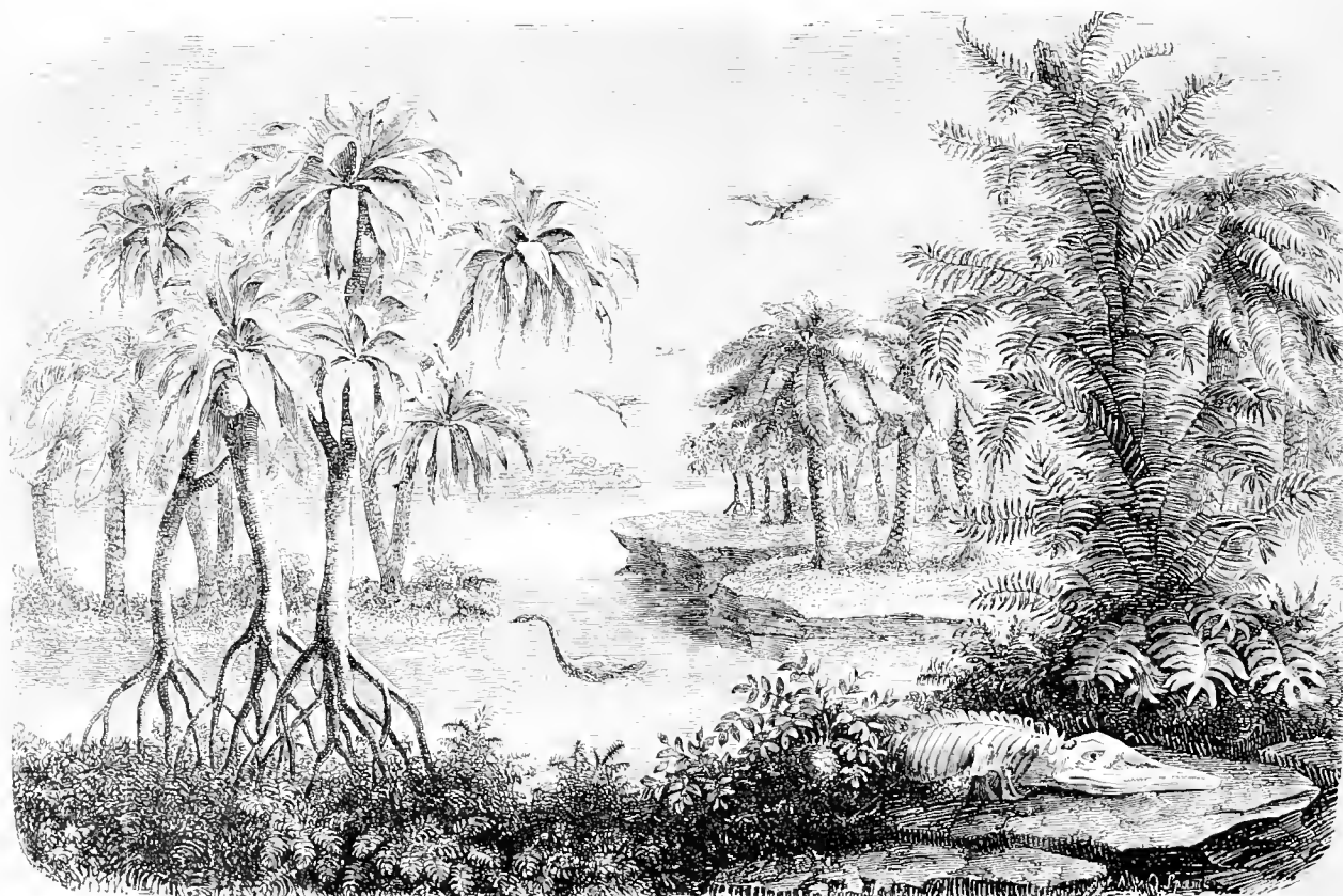
Nr. 3574 Ideale Landschaft aus der Juraformation.
