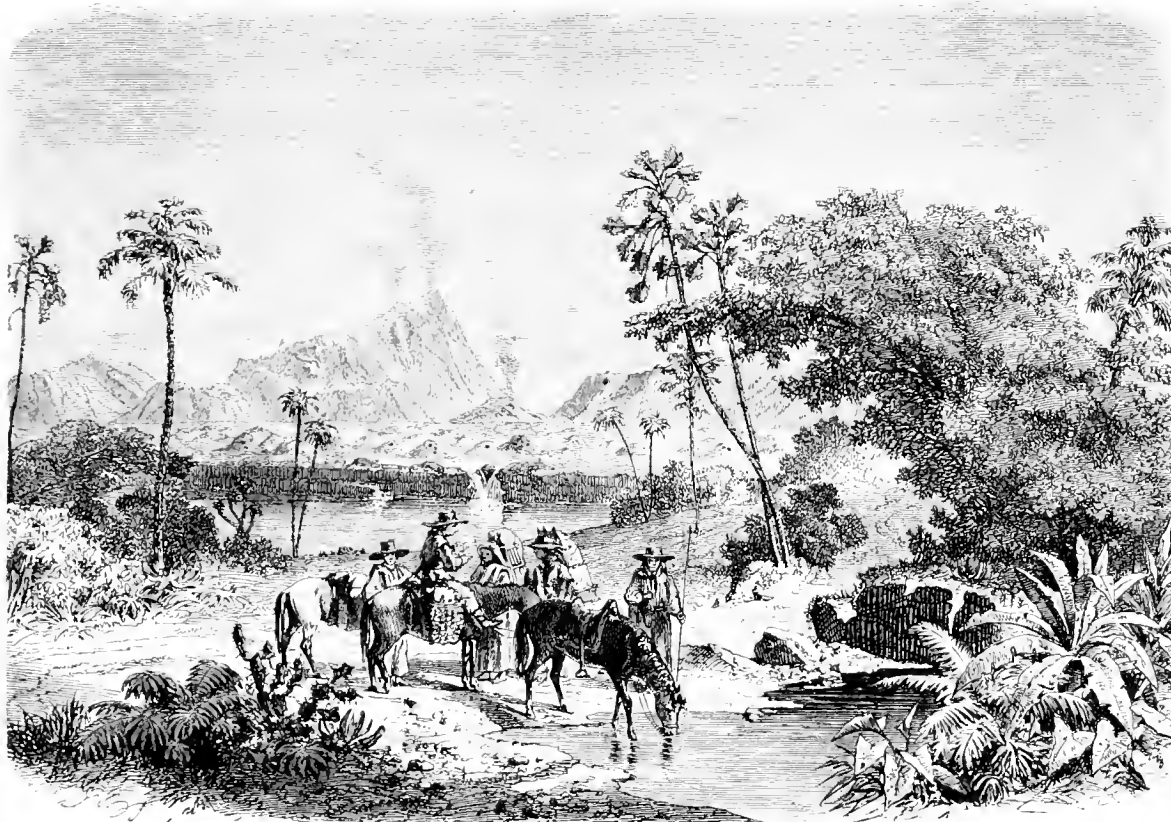
Ne. 3541. Der Vulkan Jorullo in Mexiko.
