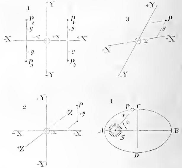
Fig. 373. Koordinatensystem.
