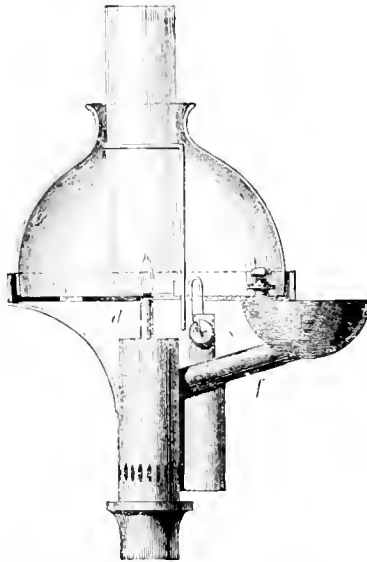
Nr. 3903 Kiosklampe mit schwimmendem Dochte.
