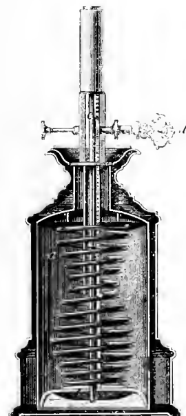
Nr. 3906 Moderatlampe.
