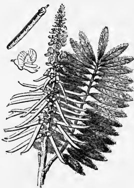
Tephrosia toxicaria.
