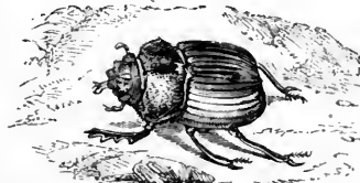
Scarabæus sacer.
