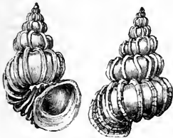
Scalaria pretiosa.
