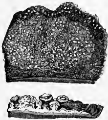
Violaria faginea.
