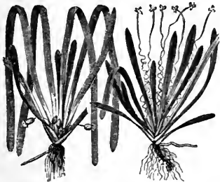
Vallisneria spiralis.
