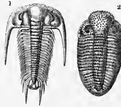
Trilobites.
