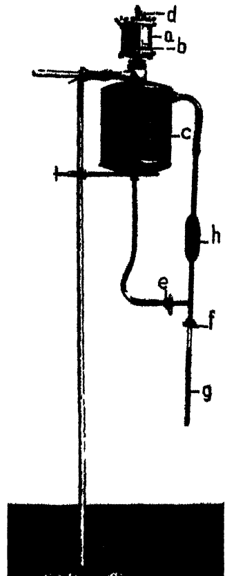
Abb. 8. Apparat zum sterilen Abfüllen des EK-Filtrates.
