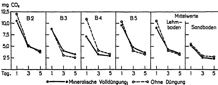
Abb. 4. Verlauf der \text{CO}_2 -Produktion des Bodens vom Lehm- und vom Sandfeld in Askov (Arbeit Christensen).
