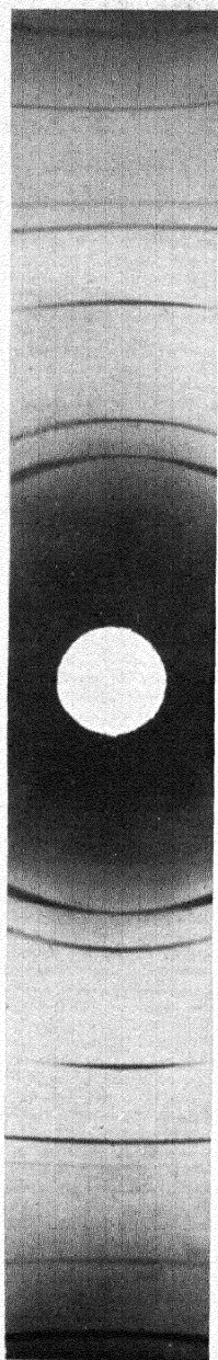
Abb. 10 Teilenaufnahme von Aluminium
