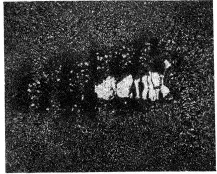
Abb. 14 Auflösung eines Schreibervites in festem Zustande nach 15 h Erhitzung auf 700° 100 \times vergrößert
