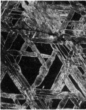
Abb. 1 Widmannstädtensche Struktur (Brückengewasser) 4 \times vergrößert
