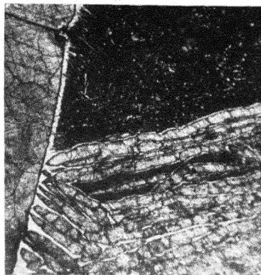
Abb. 17 Teil eines Bessitfeldes, unten normaler, oben dunkler Bessit (Bridgewater) 50 \times vergrößert
