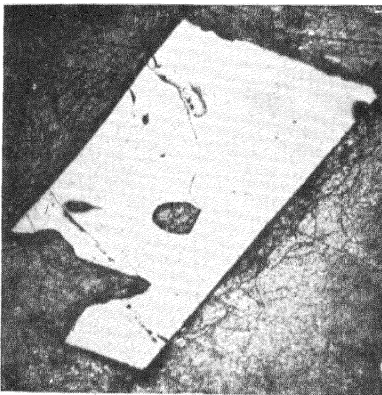
Abb. 9 Schreiberzirkonkristall 70 × vergrößert
