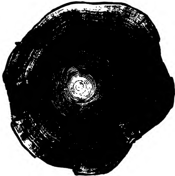
Abb. 8. Kieferscheibe mit Lachten, die durch Blaufäule fast schwarz aussehen. Dieser Pilz ist nicht in den toten Kern wegen Mangel an Nährstoffen und nicht seitlich in den nassen Splint wegen Mangel an Luft eingedrungen.
