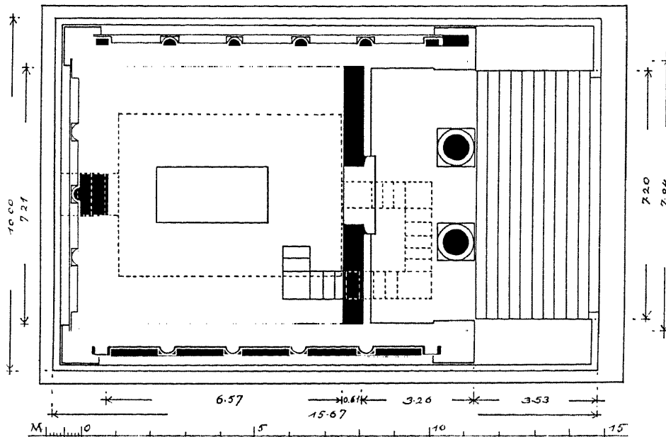
Grundriß des römischen Heroons am Westmarkt.
