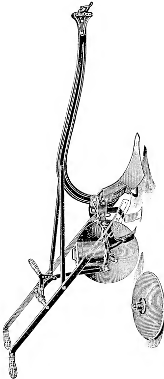
FIG. 31.--ROCK ISLAND DISK LISTER.
