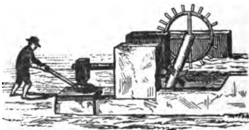
Fig. 7. Schwanzhammer mit Wasserbetrieb.
