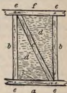
Fig. 11. Schema des Fachwerksbaus.
