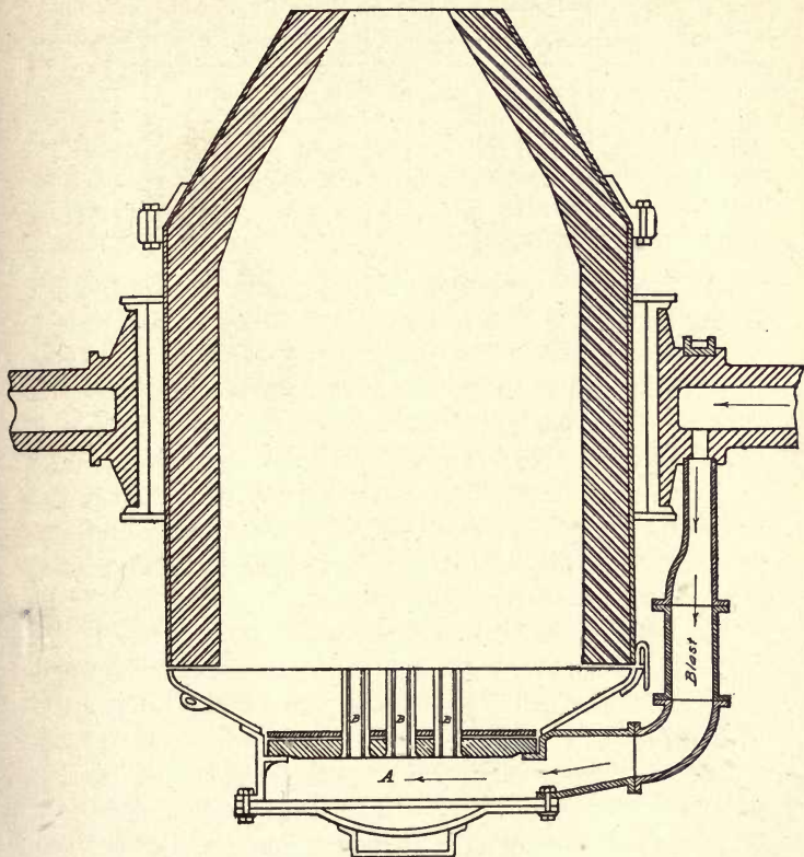
FIG. 41. Bessemer Converter.
