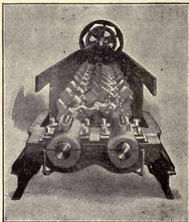
FIG. 43. Pug Mill.
