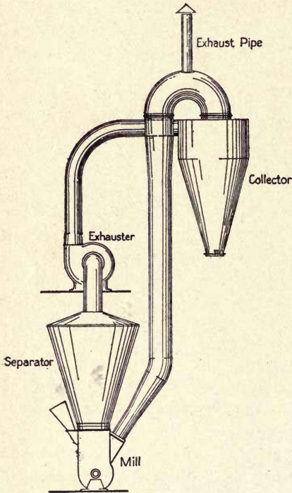
FIG. 8. Air Separator.
