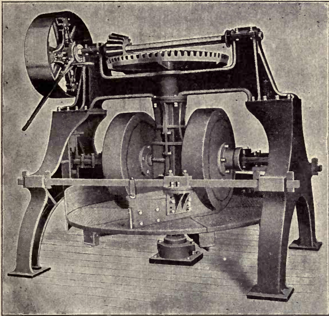
FIG. 15. Dry Pan.
