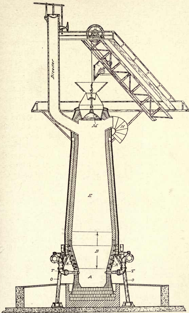
FIG. 37. Blast Furnace.
