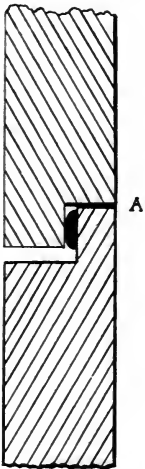
FIG. 28.—Joint in split crucible mould.
