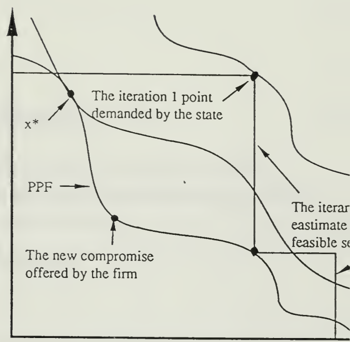
1b) Iteration 1
