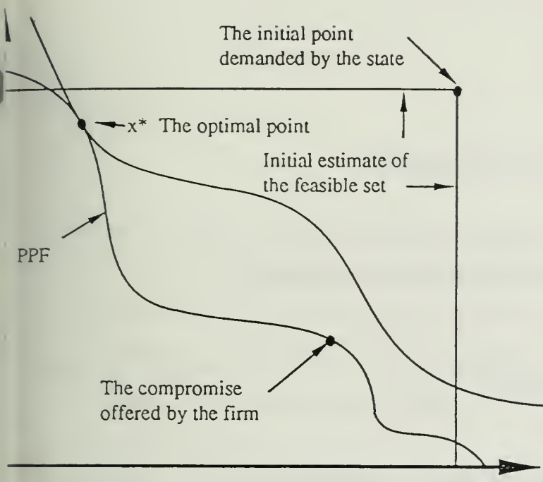
1a) Iteration 0
