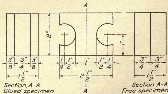
FIG. 2.—Test Specimen.
