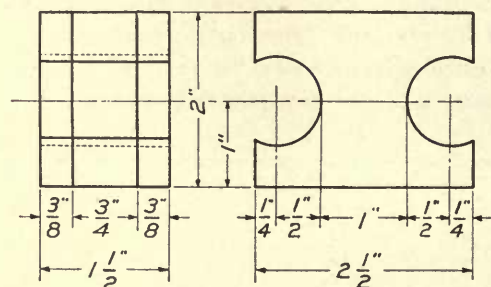
FIG. 8.—Test specimen.
