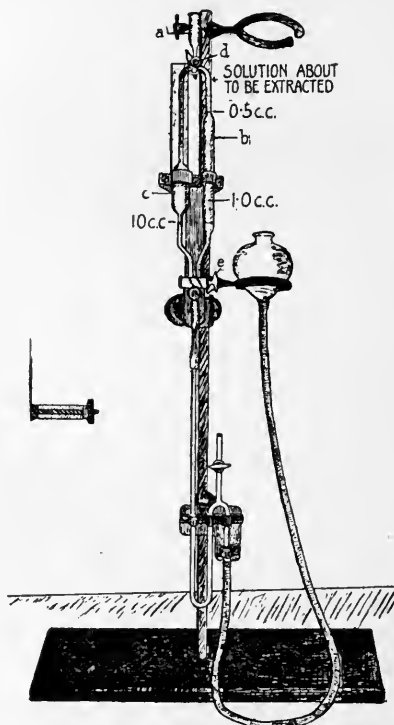
FIG. 81.—Van Slyke Micro Apparatus.
