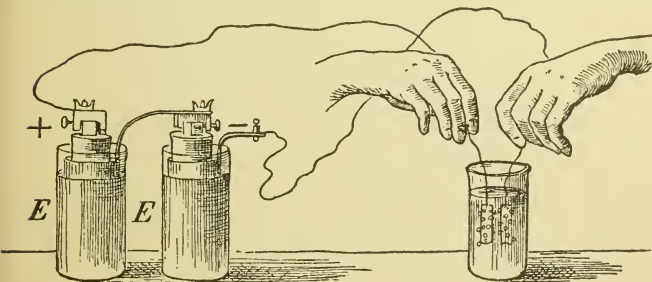
Fig. 21. Zerlegung des Wassers durch den elektrischen Strom.
