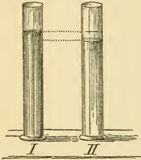
Fig. 17. Das Schmelzwasser nimmt einen geringeren Raum ein, als das Eis vorher inne hatte.
