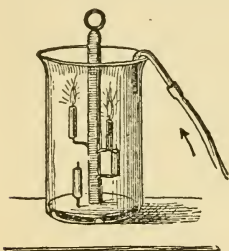
Fig. 29. Verlöschten von Kerzenflammen durch Zutönen von Kohlensäure.
