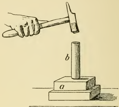
Fig. 32. Zusammenhämmern fester Kohlenensäure.
