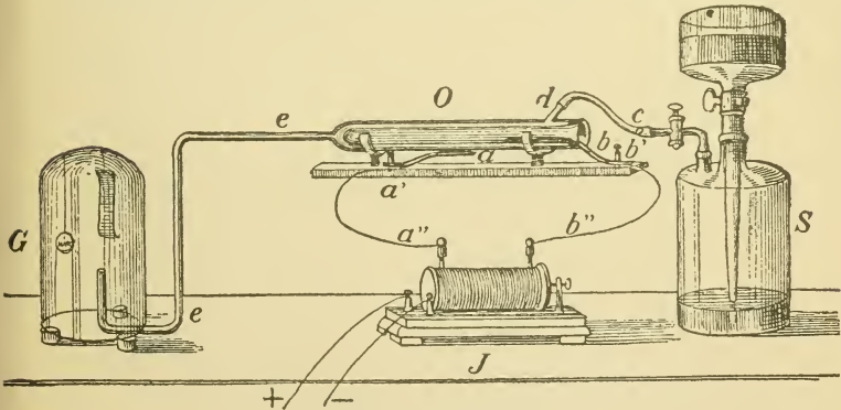
Fig. 51. Ozonapparat.
