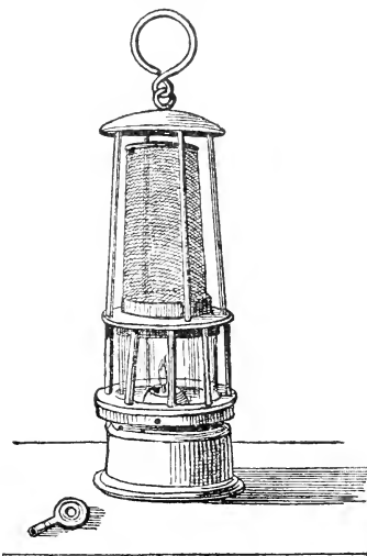
Fig. 45. Die Davy'sche Sicherheitslampe.
