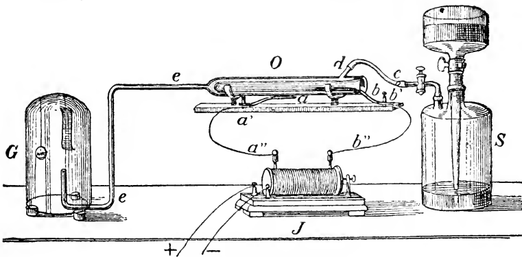
Fig. 51. Ozonapparat.
