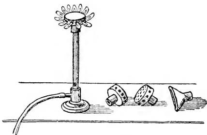
Fig. 43. Bunsen-Brenner mit seitlich durchlöcherter Luftabscheibe.
