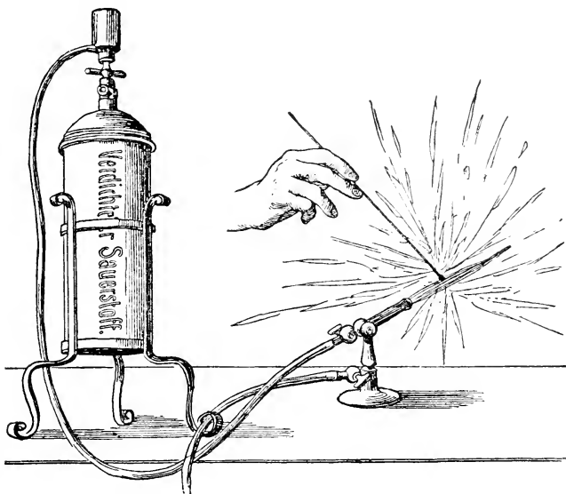
Fig. 41. Verbrennen von Eisen im Sauerstoffgebläse.
