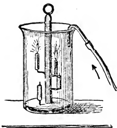
Fig. 29. Verlöschen von Kerzenflammen durch Zutönen von Kohlensäure.
