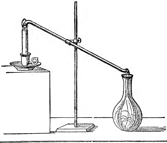
Fig. 40. Im Innern der Kerzenflamme befinden sich Dämpfe, welche sich durch ein Glasrohr ableiten lassen.
