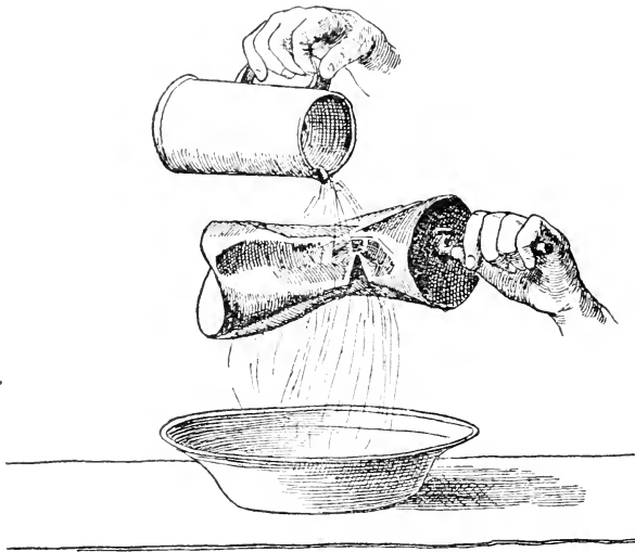
Fig. 19. Der Kessel wird in demselben Augenblick, in welchem sich der Wasserdampf infolge der Abkühlung zu flüssigem Wasser verdichtet, durch das Gewicht der Luft zusammengedrückt.
