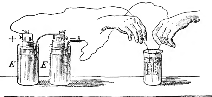
Fig. 21. Zerlegung des Wassers durch den elektrischen Strom.
