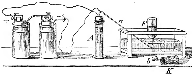
Fig. 22. Auffammeln der bei der elektrolytischen Zersetzung des Wassers entstehenden Gase.
