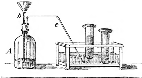
Fig. 27. Aus dem kohlensauren Kalk macht Salzsäure die Kohlensäure wieder frei.
