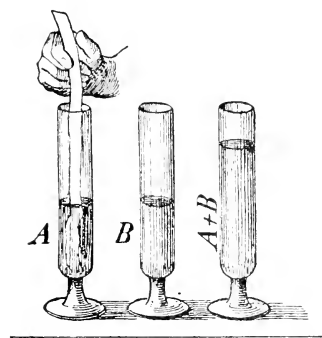
Fig. 9. Nachweis einer chemischen Reaktion mit Reagenzspapier.
