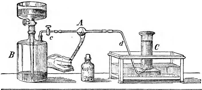
Fig. 10. Chemische Einwirkung eines Gases auf einen festen Körper.
