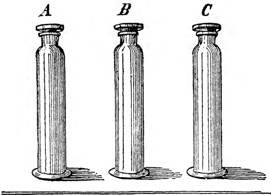
Fig. 5. Verschiedene farblose Gase.
