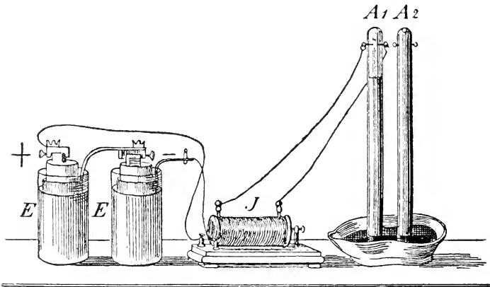
Fig. 24. Wiedervereinigung von Wasserstoff und Sauerstoff zu Wasser durch den elektrischen Funken.
