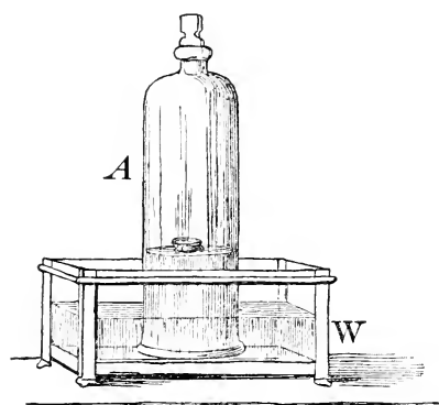
Fig. 13. Das Wasser steht innerhalb der Glocke höher, wie in der Wanne.
