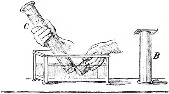
Fig. 15. Überfüllen des Sauerstoffs und Stickstoffs in den Glaszylinder C . würden alle weiteren Versuche mit dem Gemisch zu dem Ergebnis führen, daß es sich wie Luft verhält. Durch einfaches Zusammenmischen von Sauerstoff und Stickstoff erhielten wir also ein 5
