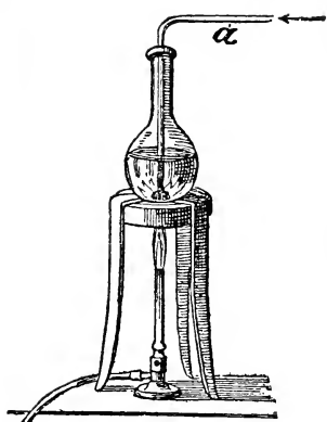
Fig. 37. Verbrennung von Phosphor unter Wasser.
