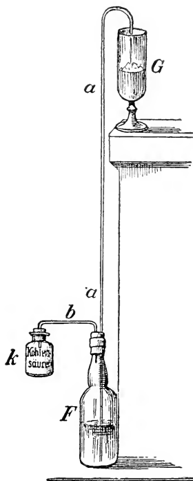
Fig. 33. Heben von Bier mittels fester (flüssiger) Kohlensäure.
