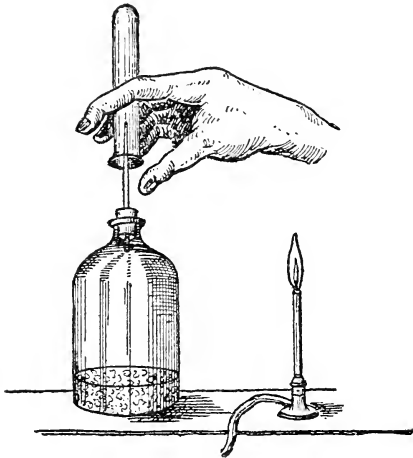
Fig. 26. Ist die Entzündung des aus der Flasche entweichenden Wasserstoffgases gefahrlos?
