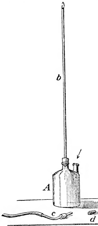
Fig. 44. Bei gesteigerter Zumischung von Luft zu Leuchtgas entsteht allmählich ein explosives Gemisch.
