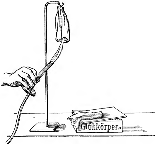
Fig. 49. Abbrennen eines Glühkörpers.
