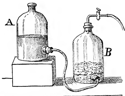
Fig. 28. Apparat zur Darstellung von Kohlensäure aus Marmor.
