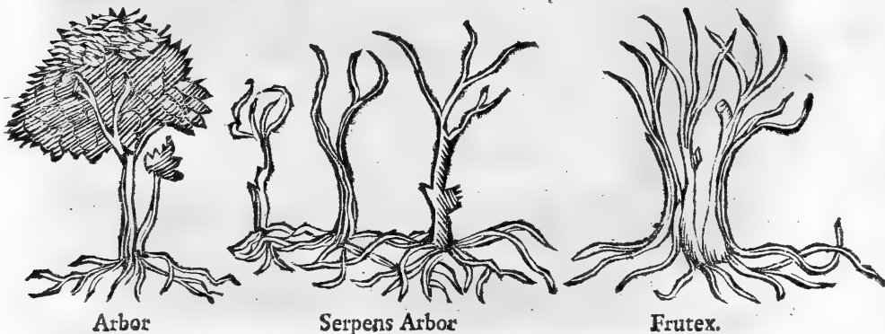
Arbor
