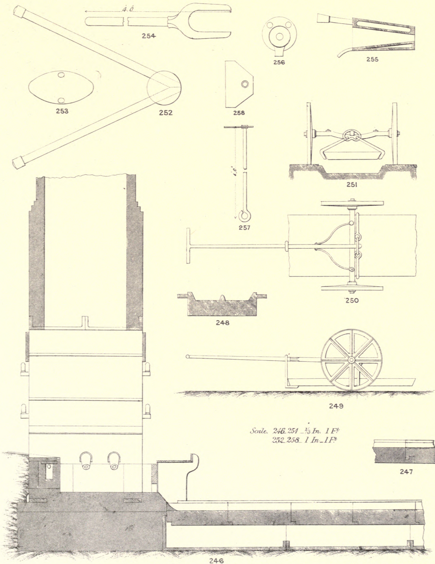
LONGITUDINAL SECTION.
