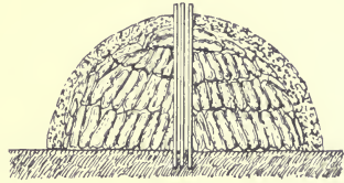
FIG. 2.—Charcoal Pile.
