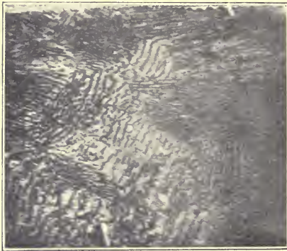
FIG. 66.—Cementite (Stead).
