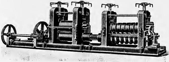
FIG. 49.—Rolls.
