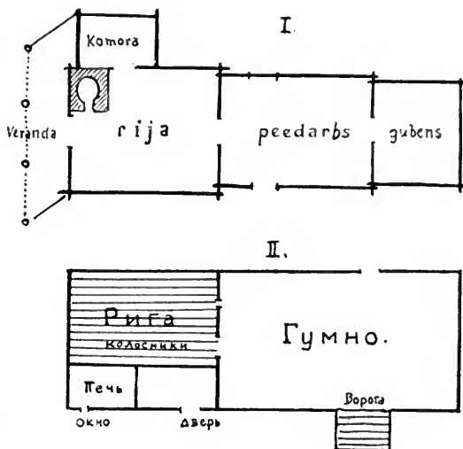
Obr. 131. I. Sušárna lotyšská z poríčí Dviny (podle Bielensteina) a II. ríga novgorodská z okolí Borovičů (podle Sinozerského).
