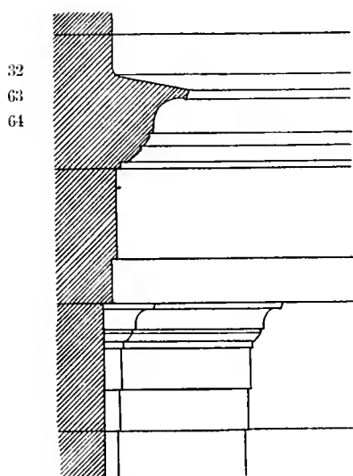
Pilasterkapitell im Innern.
