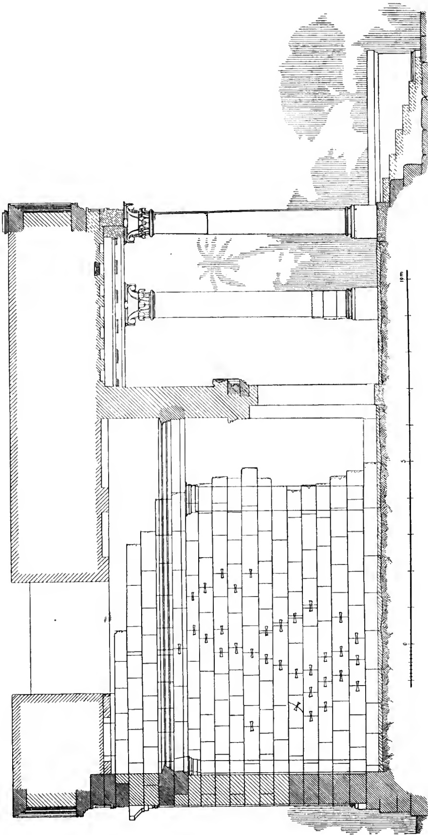
DER AUGUSTUSTEMPEL AUF PHILAE. LÄNGSSCHNITT.
