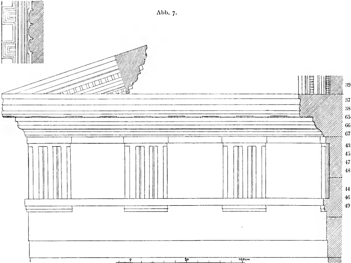
Triglyphon, Haupt- und Giebelgesims.
