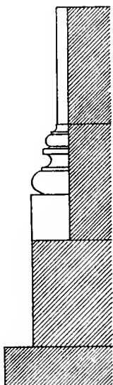
Pilasterbasis der äußeren Ecken.
