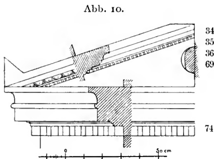
Türbegrönung.
