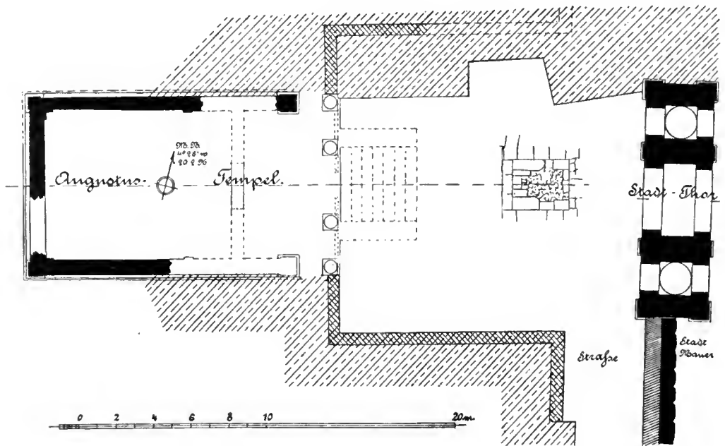
Grundriß des Tempels mit Vorplatz.
