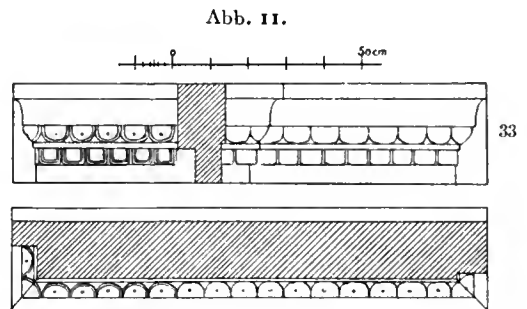
Fensterbegrönung.
