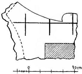
Oberlager des Antenkapitells der NW.-Ecke mit Vorzeichnung.
