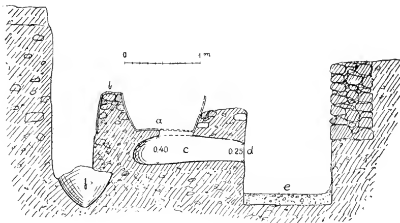
Abb. 1. Schnitt durch den Töpferofen (Tiryns).
