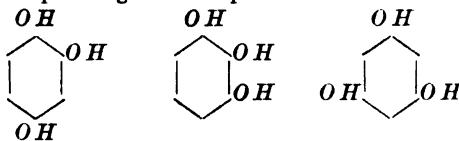
Oxyhydrochinon Pyrogallussäure Phloroglucin
