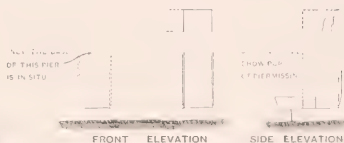
OF PIERS N. END OF S. WING
