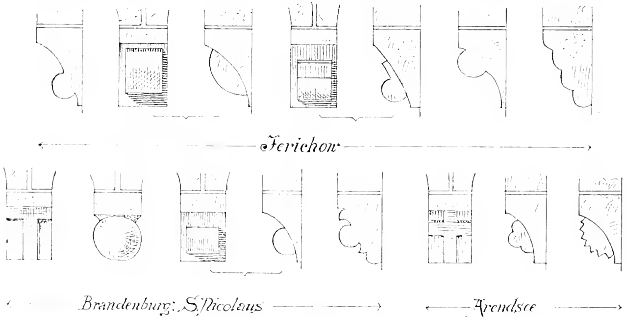
Fig. 8. Backsteinkonsolen deutscher Bauten.
