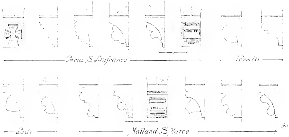
Fig. 7. Backsteinkonsolen italienischer Bauten.
