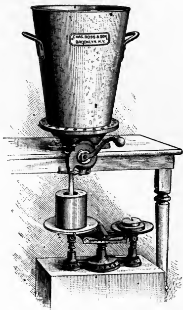
FIG. 13.—Can Filling Machine. Chas. Ross & Son Co., Brooklyn, N. Y.
