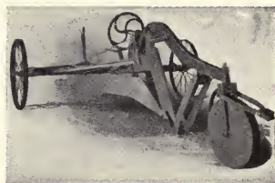
FIG. 30. Cyclone Ditcher
