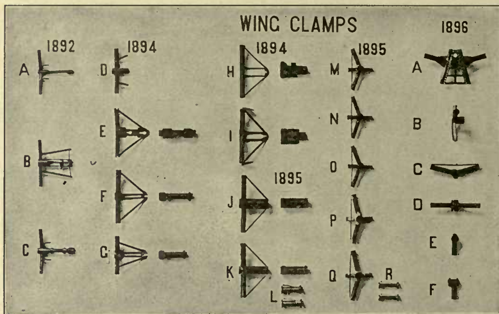
FIG. 16. Wing clamps, 1892-1896.
