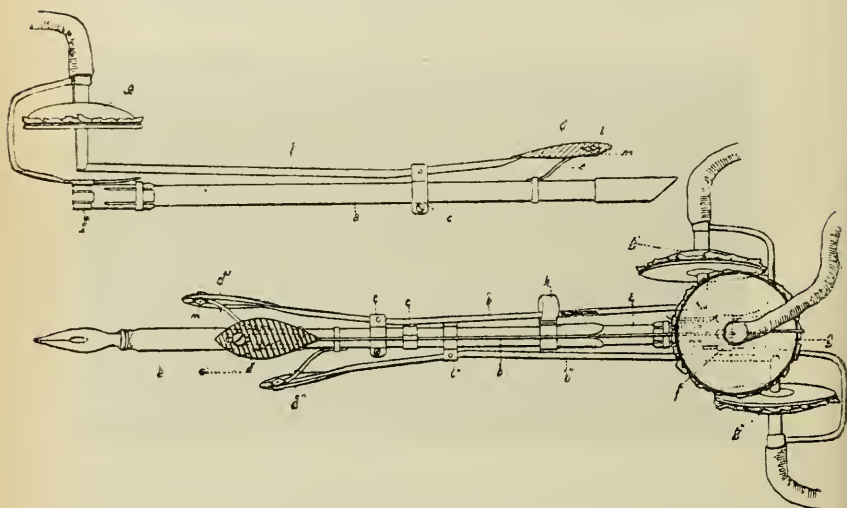
Fig. 102. — Graphographe d'Obici.
