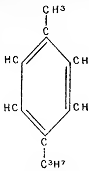
Cymène.
