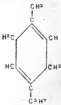
Terpène.
