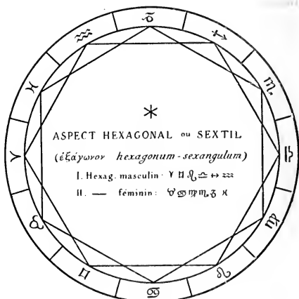
Fig. 21. Aspect sextil.
