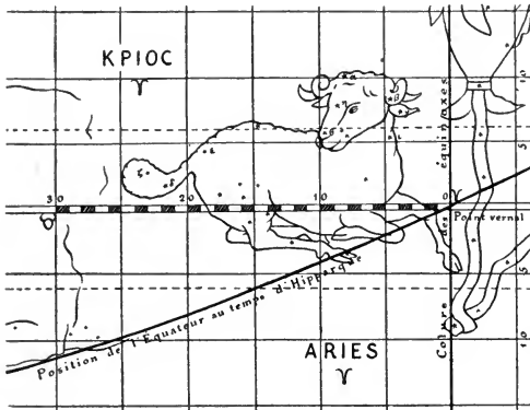
Fig. 3. Le Bélier.
