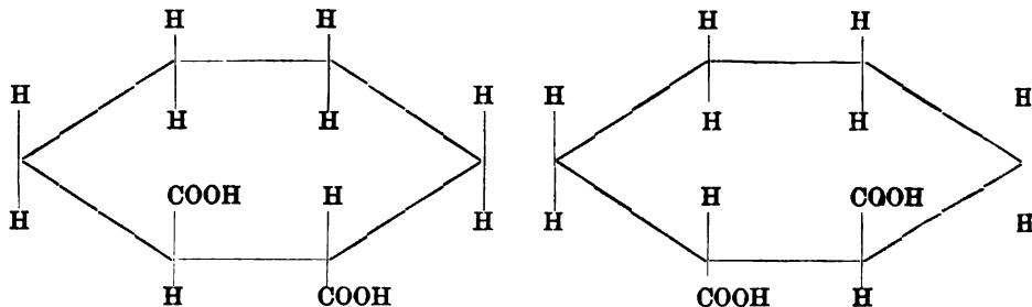
Enantiomorphe Formen der Transhexahydrophthalsäure
