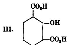
2-Oxyisophtalsäure 4 , 2-Oxybenzencarbonsäure(1.3)
