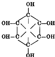
Hexaoxybenzol, S. 429
