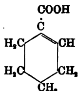
I. \Delta^1 -Tetrahydrobenzoëssäure
