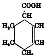
II. \Delta^2 -Tetrahydrobenzoëssäure
