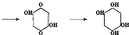
Dioxychinon (S. 452)
