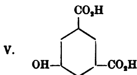
5-Oxyisophthalsäure 3 , 5-Oxybenzdicarbon- säure(1.3)
