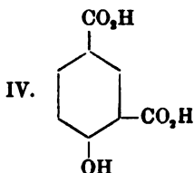
4-Oxyisophthalsäure 1,2 , 4-Oxybenzdicarbon- säure(1.3)
