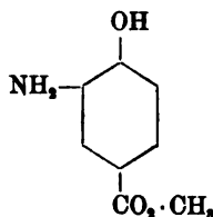
Orthoform neu (dimorph; Schmelzpunkt 110—111° bzw. 142°)
