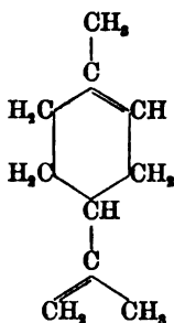
\Delta^{1,8(9)} -p-Menthadien (Dipenten)
