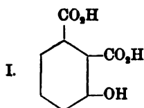
3-Oxyphtalsäure 2 , 3-Oxybenzencarbonsäure(1.2)
