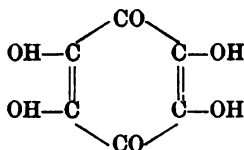
Tetraoxychinon, S. 453
