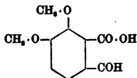
1-Methyl-3,4-Dimethoxybenzencarbonssäure (2),
