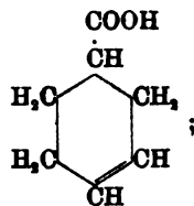
III. \Delta^3 -Tetrahydrobenzoëssäure
