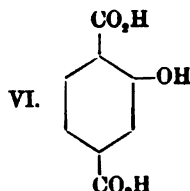
Oxyterephthalsäure 4 , 2-Oxybenzdicarbon- säure(1.4)
