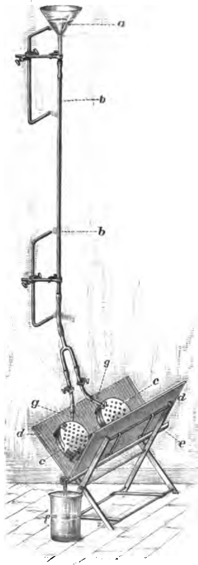
Fig. 58. HEMPEL'sche Filterpresse.
