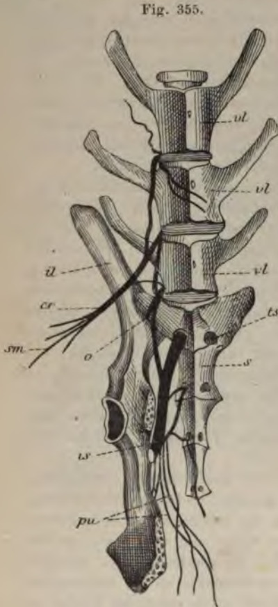
Lep. can. — Lenden- und Kreuzgeflecht (nach Krause). vl , fünfter, sechster und siebenter Lendenwirbel; s , Kreuzbein; ts , Kreuzbeinlöcher; il , Darmbein; cr , N. cruralis ; sm , N. saphenus ; o , N. obturatorius ; is , N. ischiaticus ; pu , N. pudendi in drei Bündeln vereinigt.
