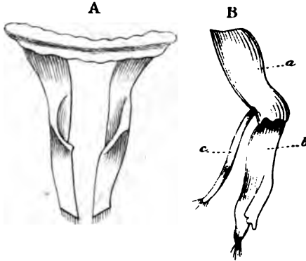
Astacus fluviatilis . — Begattungsanhänge des Männchens. A , das erste Paar mit seiner Rinne; B , ein Anhang des zweiten Paares; a , Basalglied; b , lamellöses Endglied; c , fadenförmiges Seitenglied (nach Brocchi).
