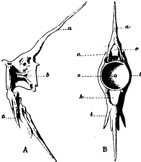
Perca fluviatilis . — Der 21. Wirbel doppelt vergrössert. A, Profil; B, von vorn. Dieselben Buchstaben. h , Haemalcanal.
