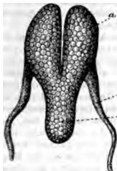
Astacus fluviatilis. — Unter der Lupe gezeichneter Eierstock. a, Vorderlappen; b, Hinterlappen; c, Eileiter.
