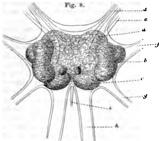
Astacus furiatilis . — Durch Glycerin aufgeklärtes Hirn, von der Rückenfläche aus gesehen (Gundlach, Oc. I, Obj. 00). a , Protocerebrum; b , Deutocerebrum; c , Tritocerebrum; d , Augennerv; e , Oculomotorius; f , Hautnerv; g , Fühlernerv; h , Schlundconnectiv; i , Hirnnerv, der nach hinten zum Magennervensystem geht. Die von der unteren Fläche des Hirns ausgehenden Antennularnerven sind nicht sichtbar.
