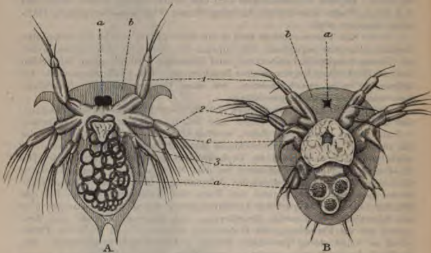
Naupliuslarven. A, von Lernaeodiscus ; B, von Cyclops ; a, unpaares Auge; b, Chitinschale; c, Oberlippe; d, Darm; 1, erstes Paar von einfachen Füßen; 2 und 3, zweites und drittes Paar zweispaltiger Ruderfüsse.
