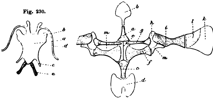
Fig. 230. — Rana esculenta . — Dreifach vergrösserter Hyoidknorpel. a , Körper; b , vordere Bogen; c , hintere Bogen; d , Griffelfortsätze; e , Thyroidhörner.
