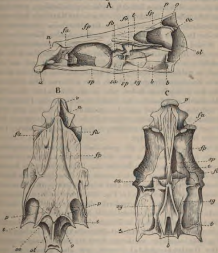
Perca fluviatilis . — Der Schädel in natürlicher Grösse. A, Profil; B, Oberseite; C, Unterseite; fo, Postfrontale; fp, Frontale; fa, Praefrontale; e, Ethmoideum; p, Parietale; b, Basilare; o, Occipitale superius; oe, Occipitale externum; ol, Occipitale laterale; sa, Orbitosphenoideum; sg, Prooticum; sp, Parasphenoideum; n, Nasale; v, Vomer; t, Temporale.
