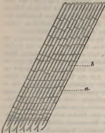
Stück des Skelettes des Kiemenkorbes. a , einfache Stäbchen; b , zweispaltige Stäbchen. (Der Kopf ist nach rechts gerichtet zu denken.)
