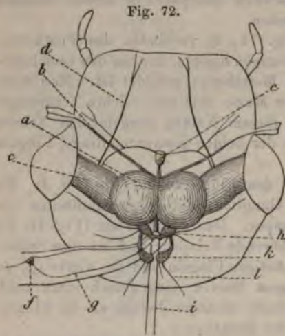
Vordertheil des Centralnervensystemes mit den verschiedenen Visceralganglien. a, Hirn; b, Fühlernerven; c, Sehnerven; d, Nerven der Oberlippe; e, Stirnganglion; f, Schlundmagenganglion; g, Aeste des rücklaufenden Nervens nach seiner Theilung; h, Herzganglien; i, davon ausgehende, längs des Rückengefässes laufende Nerven; k, l, Ganglien und Nerven der Tracheenstämme des Kopfes. (Nach Blanchard.)
