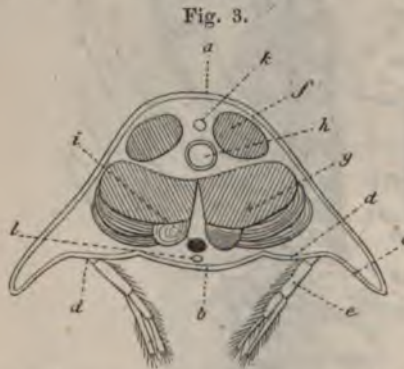
Astacus fluviatilis . — Querschnitt eines Somiten des Abdomens, welcher die allgemeine Anordnung der Organe zeigt (schematische Figur). a , Tergum; b , Sternum; c , Pleuron; d , Epimer; e , Anhang; f , Streckmuskeln des Abdomens; g , Beugemuskeln; h , Darm; i , Nervenganglion; k , obere Baucharterie; l , untere Baucharterie.
