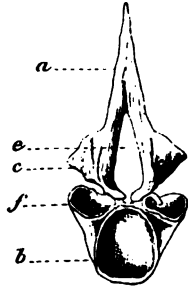
Perca fluviatilis . Der Atlas von vorn gesehen. Zweifache Vergrösserung. Dieselben Buchstaben, f , Gelenkhöhlen.
