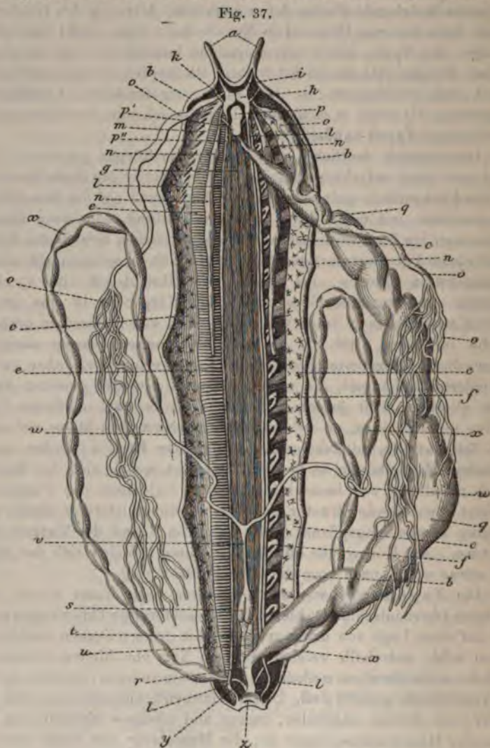
Peripatus capensis . — Die Tegumente sind längs der dorsalen Mittellinie aufgeschlitzt und die Organe auf beiden Seiten ausgebreitet worden, um die innere Bauchfläche zu zeigen (nach Moseley). Man sieht das Hirn mit den zwei seitlichen Nerven-
