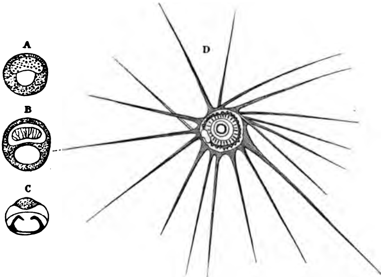
Astacus furcatus . — A, B, C, Spermatozoïden in verschiedenen Entwicklungsstadien; D, ein vollständig reifes Spermatozoid, 650 mal vergrössert (nach C. Grobben).
