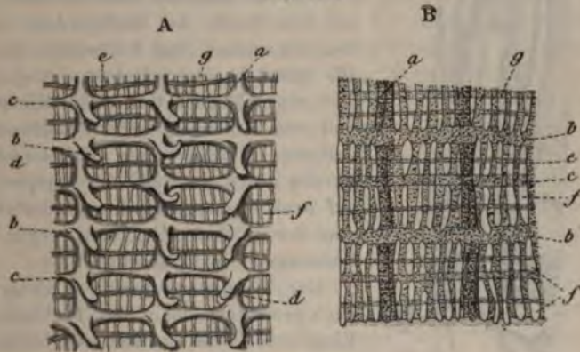
Ciona intestinalis . — Structur der Kiemenwand. A, Ansicht von innen, B, von aussen. Gundlach, Obj. 0. Camera clara. a, Längscanäle; b, Quercanäle erster Ordnung; c, Quercanäle zweiter Ordnung; d, warzenförmige Vorsprünge in die Kiemenhöhle; e, Quercanäle dritter Ordnung; f, Kiemenpalten.
