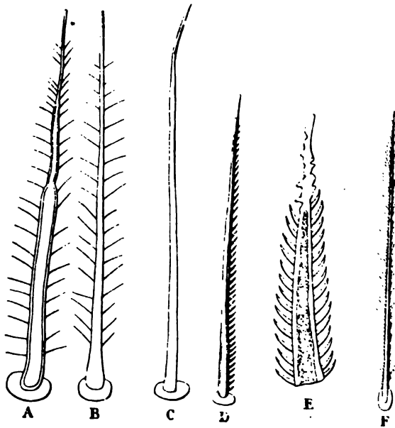
Astacus fluviatilis . — Haare der Cuticula auf verschiedenen Körpertheilen. A und B, vom Saume der Schwanzplättchen; C, vom Ende des dritten Paares der Kieferfüsse; D, Gräte der Kieferfüsse; E, die gleiche unter stärkerer Vergrösserung; F, Haar an der Basis der Antennulen.
