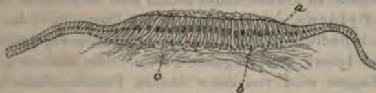
Querschnitt einer Hörleiste. Verick, Oc. 3, Obj. 2. Camera clara. a , lange Sinneszellen; b , Stützzellen; c , Nervenendigung.
