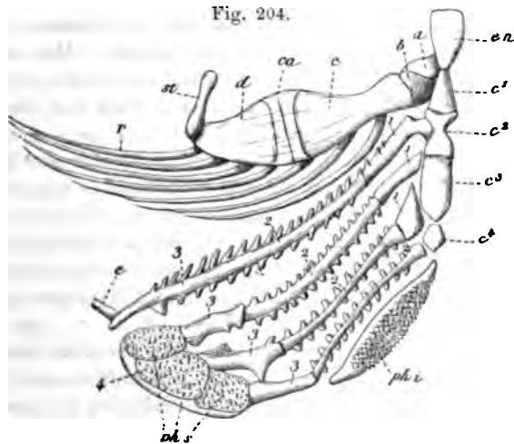
Perca fluviatilis . — Die eine Hälfte der Kiem- und Zungenbeinbogen ausgebreitet und von der inneren Fläche gesehen. Natürliche Grösse. en , Entoglossum; a , b , Gelenkstücke des seitlichen Schenkels des Zungenbogens; c , d , abgeplattete Stücke desselben Bogens; ca , knorpeliges Verbindungsstück derselben; c , stabförmiges Verbindungsstück zwischen dem ersten Kiemebogen und dem Schädel; 1, unteres; 2, mittleres; 3, oberes Stück des Bogens; st , Griffelbein; r , Kiemenhautstrahlen; phs , obere Schlundknochen; phs , untere Schlundknochen; 4, zahntragende Stücke derselben; c 1 bis c 4 , Copulae.
