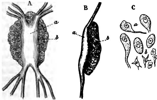
Ciona intestinalis . — Centralganglion und Untergangliendrüse. A, von oben; B, von der rechten Seite. a, Ganglion; b, Drüse. C, Isolirte Nervenzellen. a, der Peripherie; b, Sternzellen aus der Mitte des Ganglions (Gundlach, Oc. 1, Obj. 5).
