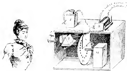
Fig. 1. — Principe de l'appareil de M. Dussaud pour essais de transmission des images à distance. — Transmetteur.
