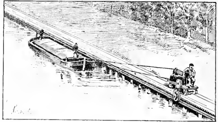
Fig. 10. — Halage des bateaux sur les canaux au moyen d'un tracteur électrique à crémaillère.
