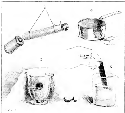
Fig. 4. — Liquefaction de l'air.
