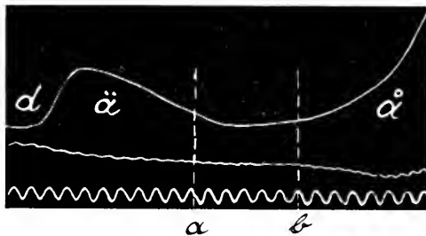
Fig. 6. dä ästäl . Oben orale lautstromkurve, in der mitte stimmungskurve, unten zeitkurve ( 1/100 sek.). Die kurven sind etwas vor beginn der s -enge abgeschnitten. Zwischen den senkrechten gestrichelten linien a und b der kelpkopf-»verschlusslaut«, während dessen die stimmbänder mit geringerer amplitude, aber in (wenigstens im original) regelmässiger weise weiterschwingen. Vergr. 1 : 1.
