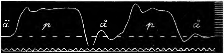
Fig. 9. dä päpā . Atemdruck im mundinnern hinter den lippen während des anlautenden und inlautenden p . Die gestrichelte linie (= nulllinie für den atemdruck) ist nachträglich gezogen. Unten zeitkurve ( \frac{1}{100} sek.). Rechts skala zur bestimmung des absoluten masses der drucksteigerung im mundinnern; der abstand zwischen zwei benachbarten strichen entspricht dem druck einer wassersäule von 10 mm. Vergr. 1 : 1.
