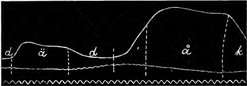
Fig. 5. dä d'äk . Kurvenanordnung wie oben. Nach aufhebung des d -verschlusses steigt hier die lautstromkurve zuerst ser langsam, dann etwas stärker, während gleichzeitig die schwingungen in der stimmkurve eine amplitude zeigen, die nur wenig geringer ist als während des d -verschlusses. An das d schliesst sich offenbar zunächst ein z -artiger laut an. Die amplitude der stümschwingungen nimmt dann ziemlich unvermittelt (bei beginn des eigentlichen ä ) ab. Bei der reproduktion sind die in wirklichkeit ser deutlichen und regelmässigen, wenn auch niedrigen schwingungen in der stimmkurve für ä zum grössten teil verloren gegangen. Vergr. 1 : 1.
