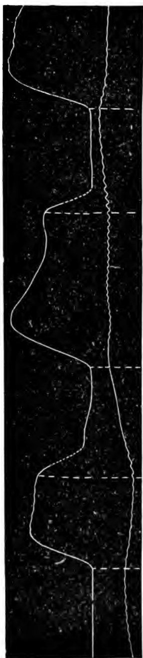
Fig. 1. dä kid . Oben kurve des oralen lautstroms, unten stimmbandkurve. Die senkrechten gestrichelten linien sind nachträglich gezogen und bezeichnen die grenzen der einzelnen laute. Bei a aufhebung des d -verschlusses von dä ; schon vorher, also während des d -verschlusses, stimmbandschwingungen. a—b dauer des ä . Bei b ist der k -verschluss vollzogen; im anfangsteil des verschlusses noch stimmbandschwingungen. Bei c aufhebung des k -verschlusses; die stimmbandschwingungen setzen erst eine beträchtliche zeit nach c ein. Bei d ist der verschluss des d von kid vollzogen, bei c aufhebung dieses verschlusses; die stimmbandschwingungen, die den verschluss ausfüllen, dauern auch noch eine lange zeit nach aufhebung des d -verschlusses an. — Vergr. \frac{1}{1} . Zeit: 100 mm = 0,35 sek.
