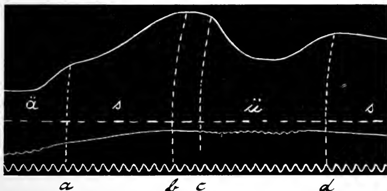
Fig. 7. dä süs . Oben orale lautstromkurve, in der mitte stimmkurve, unten zeitkurve ( 1/100 sek.). Die kurven beginnen nach dem ersten drittel des ä und sind etwa in der mitte des zweiten s abgeschnitten. Die enge des anlautenden s ist in dem durch die gestrichelte linie a bezeichneten zeitpunkt vollzogen und dauert bis zur gestr. linie b . Zwischen b und c der stimmlose abbauch des s zu ü hin. Die enge des auslautenden s ist in d vollzogen. Vergr. 1 : 1.
