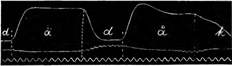
Fig. 4. dä däk . Oben orale lautstromkurve, in der mitte stimmkurve, unten zeitkurve ( \frac{1}{100} sek.). Die explosionskurve für das d von däk ziemlich steil. Sofort nach aufhebung des d -verschlusses nimmt die amplitude der schwingungen 2 in der stimmkurve beträchtlich ab. Vergr. 1 : 1.
