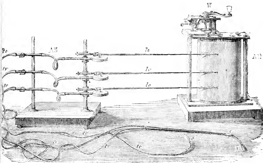
FIG. 67. — Appareil enregistreur.
