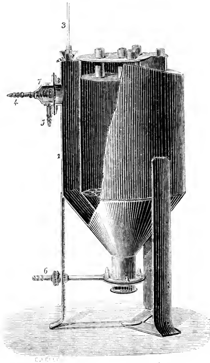
FIG. 106. — Appareil de Arsonval pour obtenir une température constante.
