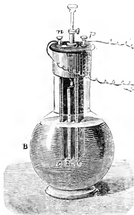
FIG. 70. — Pile de Grenet.
