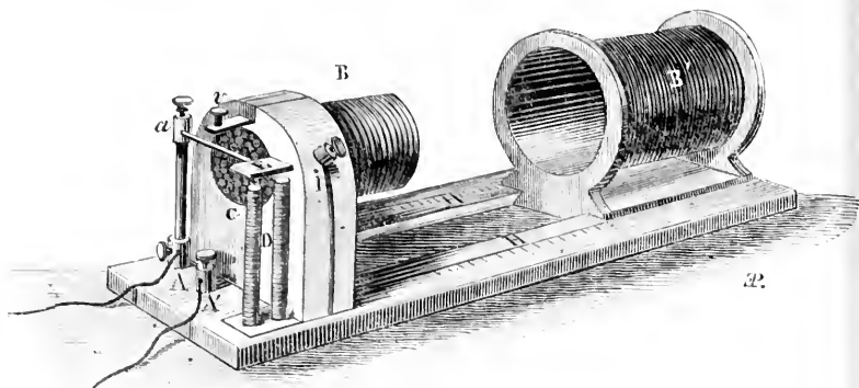
FIG. 71. — Appareil volta-faradique de Du Bois-Reymond
