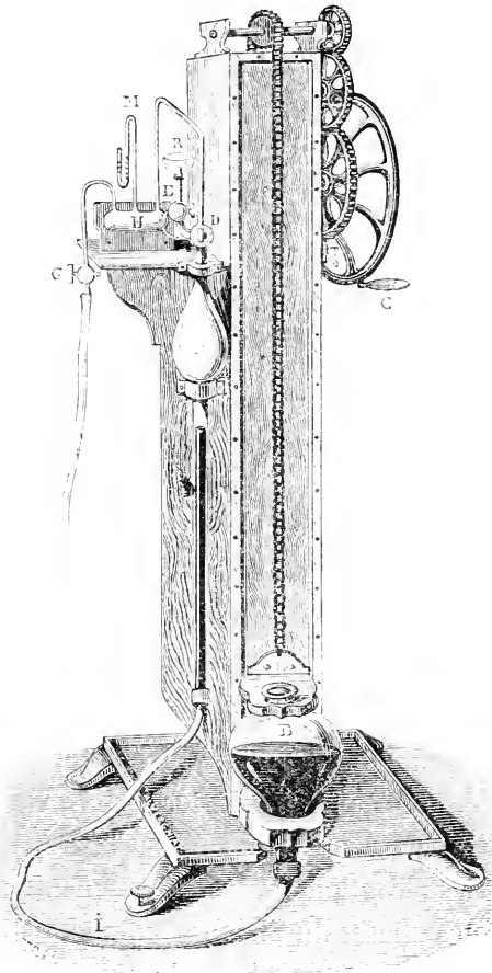
FIG. 66 - Pompe à mercure.
