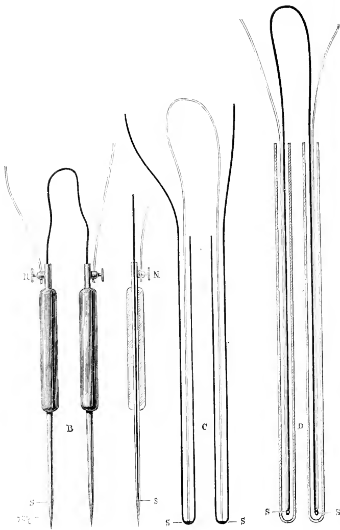
FIG. 101. — Sondes thermo-électriques de d'Arsonval.
