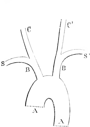
FIG. 74. — Taupe, Chauve-souris.
