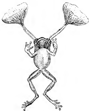
Fig. 42. — Nototrema cornutum , jeune retiré de la poche dorsale, montrant les branchies campaniformes.
