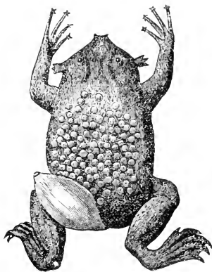
Fig. 39.— Pipa americana , femelle, avec l'ovipositeur, d'après BARTLETT.
