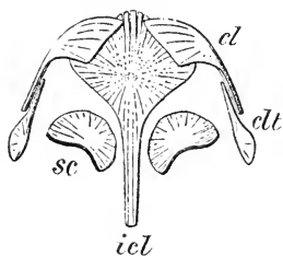
Fig. 9. — Ceinture pectorale de Discosaurus , d'après GEGENBAUR.
