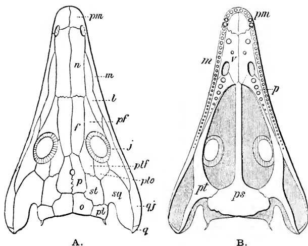
Fig. 3. — Crâne de Archegosaurus Decheni , en dessus (A) et en dessous (B). Contours d'après CREDNER
