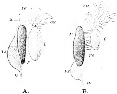
Fig. 21. — Organes génito-urinaires d'Anoures mâles.
