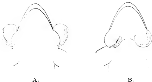
Fig. 24.— Sacs vocaux gonflés de Rana esculenta (A) et R. temporaria (B).
