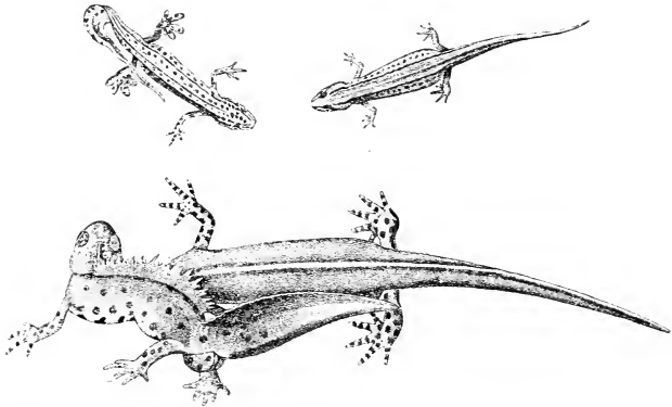
Fig. 29. — Préludes de la fécondation chez Molge vulgaris et M. cristata . D'après RUSCOXI.
