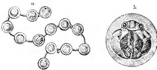
Fig. 44.— Mantophryne robusta ; a. chapelet d'œufs, b. embryon dans l'œuf. D'après L. v. MEHELY.
