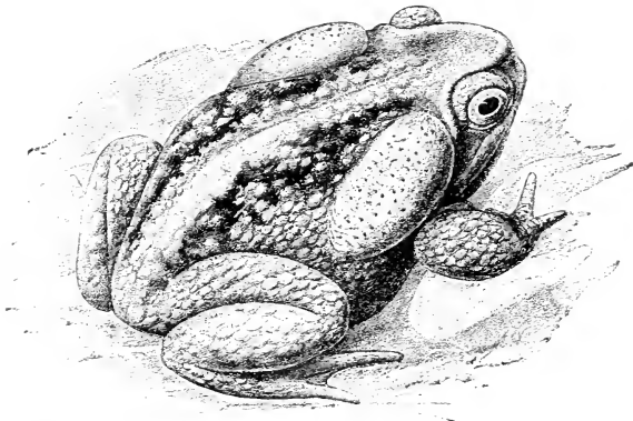
Fig. 23. — Crapaud aqua de l'Amérique du Sud ( Bufo marinus ) remarquable pour l'énorme développement des glandes à venin dites parotides.
