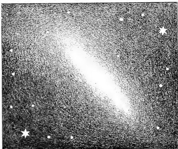
Fig. 5. — Etat que dut présenter la Terre, lorsqu'elle se condensa et passa à l'état stellaire.
