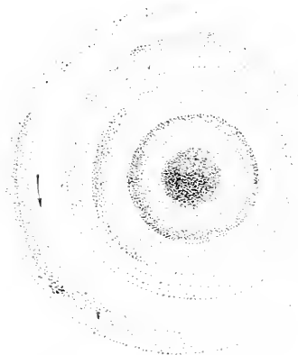
Fig. 1. — Nébuleuse de Laplace, vue par le pôle. Au milieu, le noyau très concentré du soleil. Tout autour, les anneaux d'où naissent les planètes.
