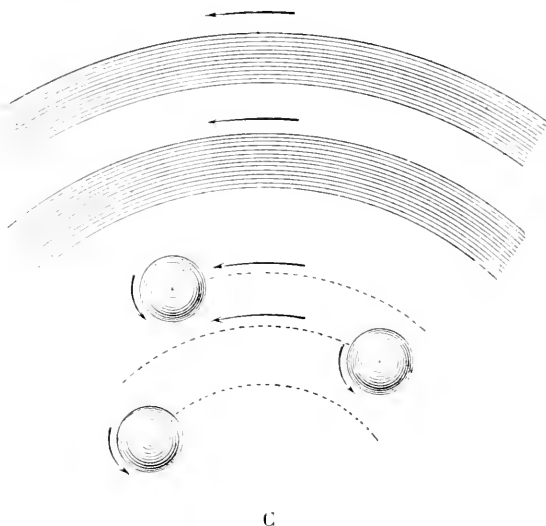
Fig. 6. — D'après M. Faye, les planètes inférieures sont formées avant les planètes supérieures.
