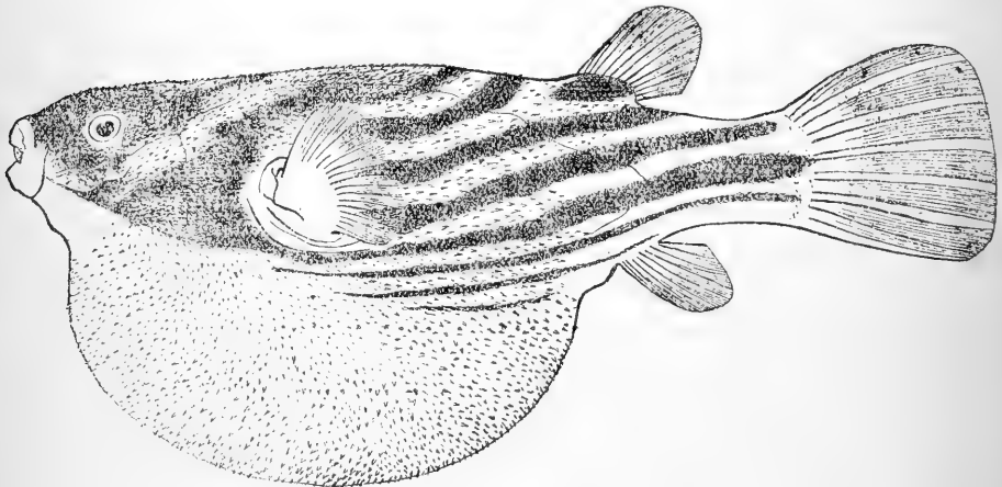
FIG. 76. — Tetradon fahaka Linné.
