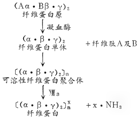
图70 尖吻蝮纤维蛋白形成过程
