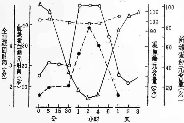
图68 尖吻蝾毒TLE对全血凝固时间 (O—O), 血浆凝血酶元时间 (●…●), 凝血酶元含量 (□…□) 及纤维蛋白元含量 (△—△) 的影响
