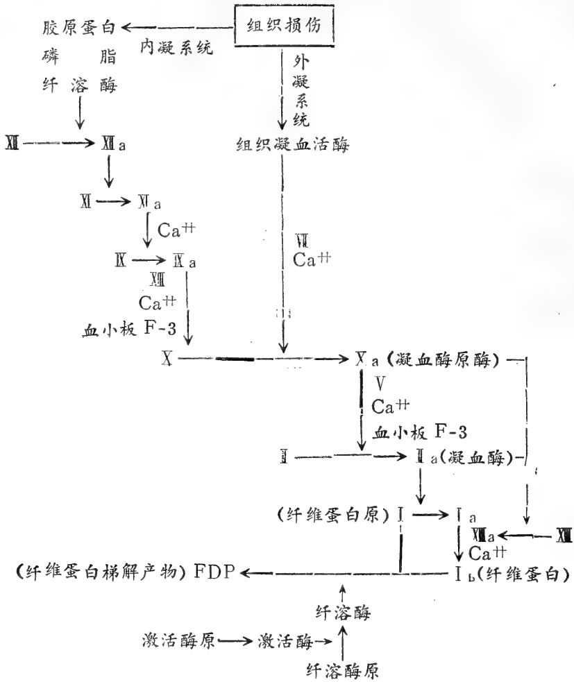
图69 尖吻蝮血液凝固过程示意图
