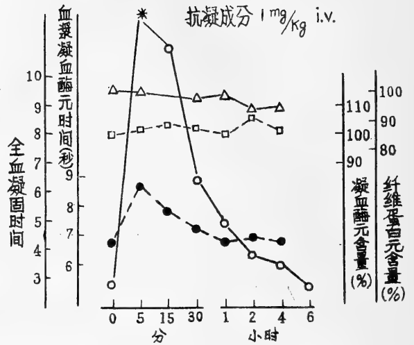
图67 尖吻蝥毒抗凝成分对全血凝固时间(○—○),血浆凝血酶元时间(○…○),凝血酶元含量(●…●)及纤维蛋白元含量(△—△)的影响。*表示全血凝固时间>6小时<24小时
