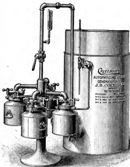
FIG: 27. The "Criterion" Generator.
