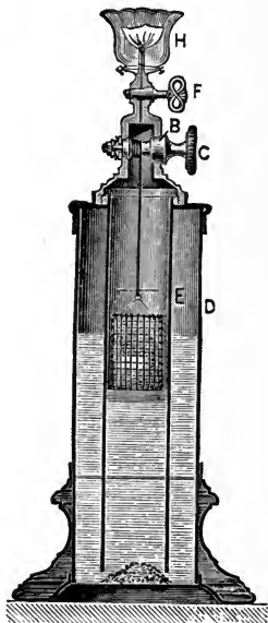
FIG. 47. Türr Lamp.
