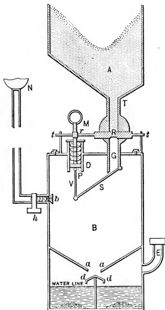
FIG. 32. Marechal Generator.
