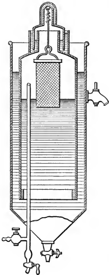
FIG. 29. d'Arsonval Generator.
