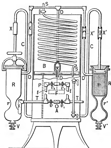
FIG. 18. Exley Generator.
