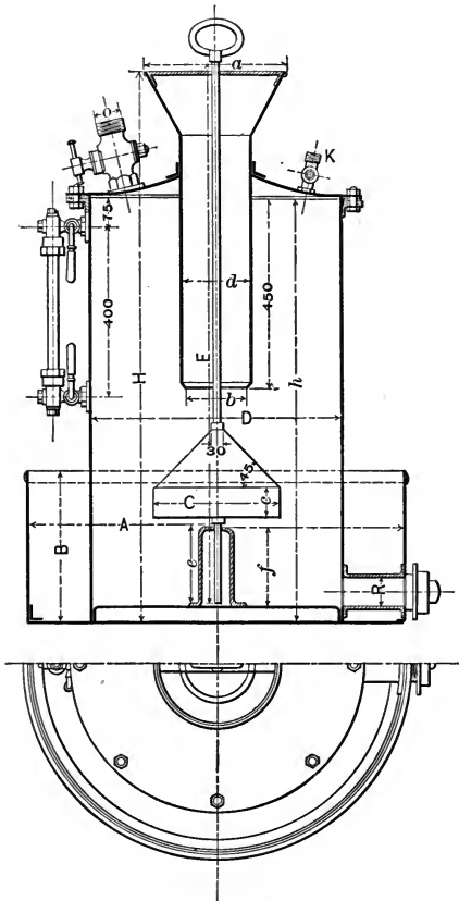
FIG. 39. Société le Gaz Acetylene.
