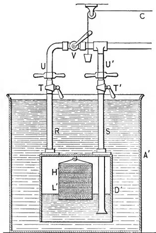
FIG. 30. Gabe Generator.
