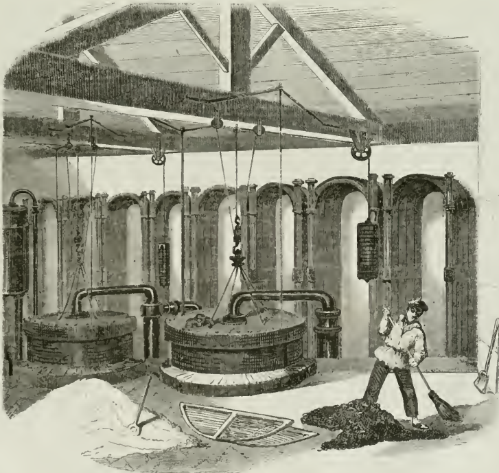
(Fabrication du Gaz. — Atelier d'épuration.)
