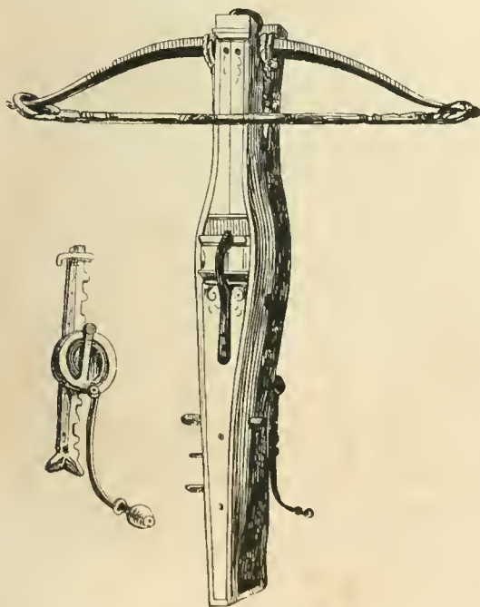
(Arbalète à cric.)
