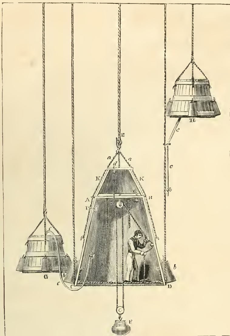
(La Cloche à Plongeur.)
